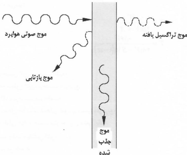
شکل ۱-۱۸-۳-۳: تراگیسیل صدای هوابرد از طریق یک جداکننده
