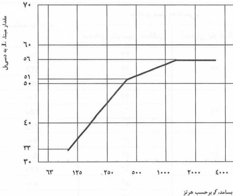
شکل ۱۸-۱-۳-۴: نمودار مقادیر مینا برای صدای هواپرد، در بندهای یک‌سوم هنگامی
